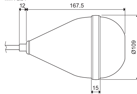
Тип 72.B1
