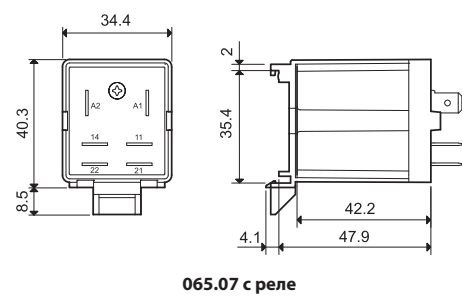
065.07 с реле
