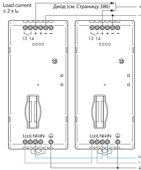
Параллельное подключение
