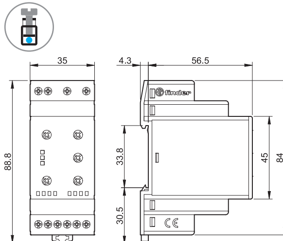
70.62 Винтовые клеммы
