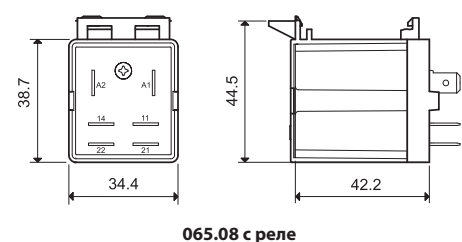
065.08 с реле
