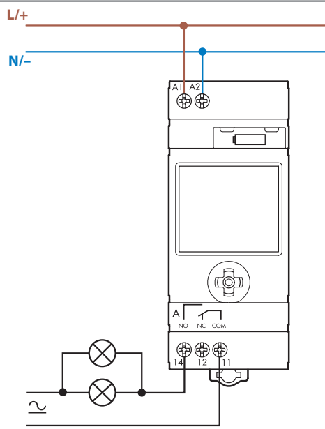
Тип 12.61 12.A1
