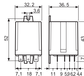
Тип 60.63
