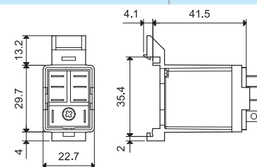
056.27 с реле
