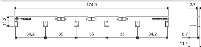
6-полюсная перемычка для Тип 22.34, ширина 35 мм 022.26 (синий) Номинальные значения 10 А - 250 В
