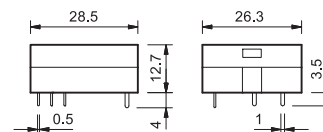
Тип 40.11 (страница 31)
