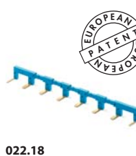
8-полюсная перемычка для Тип 22.32, ширина 17,5 мм 022.18 (синий) Номинальные значения 10 А - 250 В
