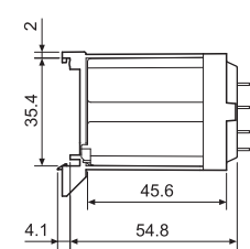
062.07 с реле
