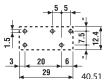
Вид со стороны выводов
