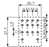
Вид со стороны выводов
