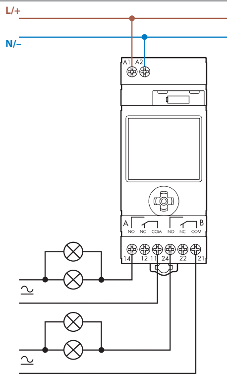
Тип 12.62 12.A2
