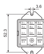
062.05 с реле
