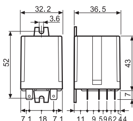
Тип 60.62
